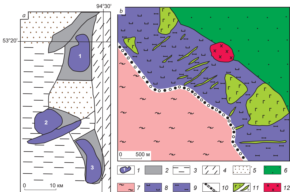
Рис. 1. Схемы геологического строения Куртушибинского офиолитового пояса Западного Саяна [4] (а), Кызыр-Бурлюкского массива [13] (б):
